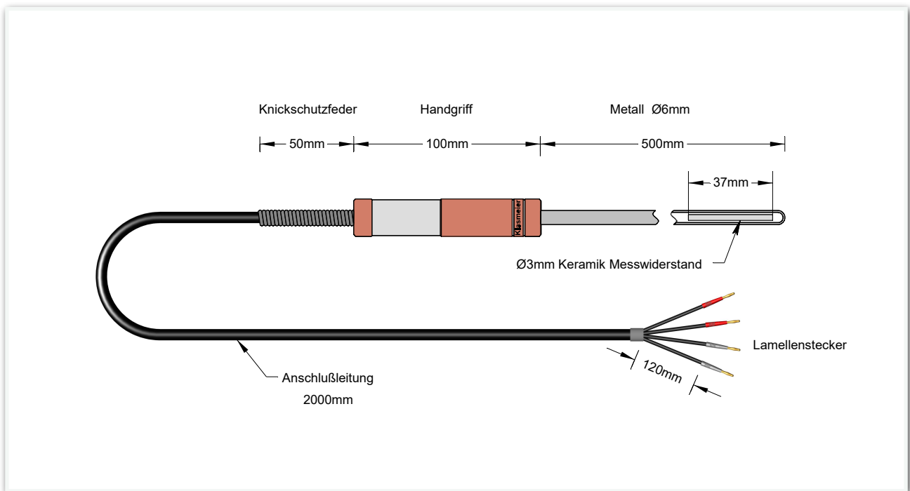
Technische Zeichnung SPRT Modell 216
